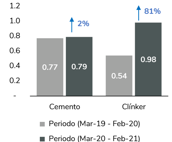
Importación anual (Millones de toneladas)
