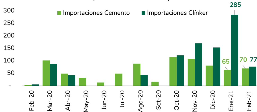
Importación mensual de cemento y clínker (Miles de toneladas)
